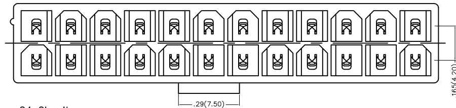
24 Circuits
